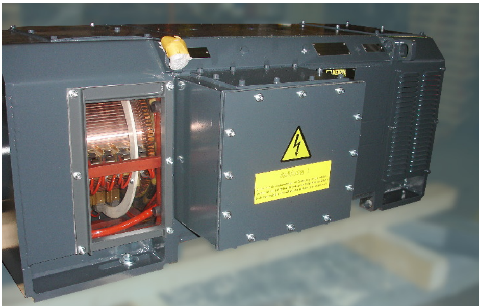
Bild: Zwei in einem: Diese speziell modifizierte, kostensparende Reservelösung von Menzel Elektromotoren ersetzt bei Bedarf zwei unterschiedliche Extruderantriebe
